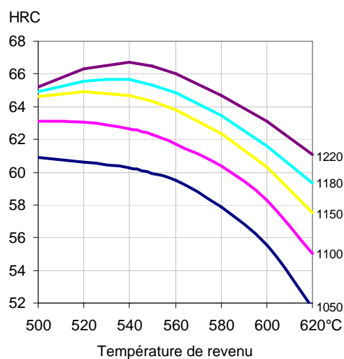
Dureté après austénitisation, trempe et revenu 2 x 1 heure
